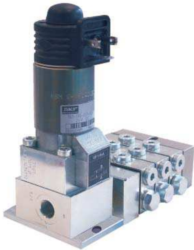
Mit 2/2-Wegemagnetventil
